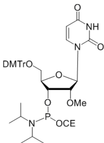
wzór strukturalny
